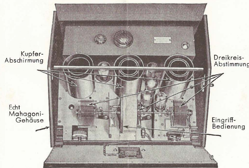
Telefunken 9, geöffnet
